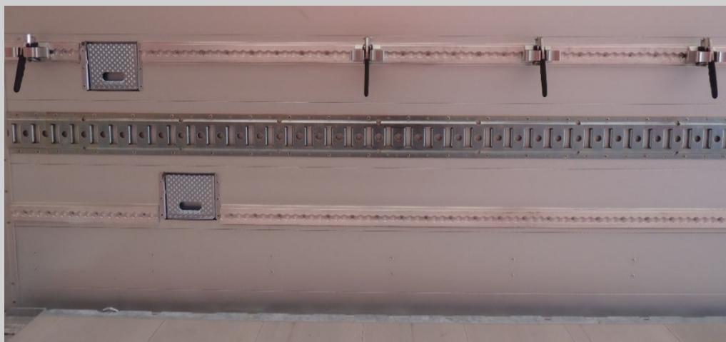
Bordwand mit Klemmen-Sicherung auf Airline-Schiene, Combianker-Schiene, Klapptritte, Zurrpunkte längs im Boden
